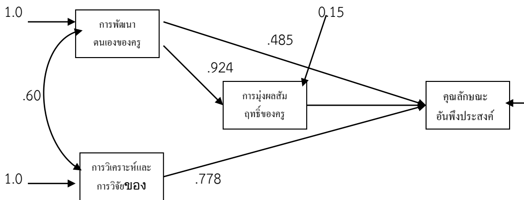
ภาพที่ 1 เส้นทางระหว่างค่าตัวแปรต้นกับตัวแปรตาม แบบ Path Analysis with LISREL (PAL)
